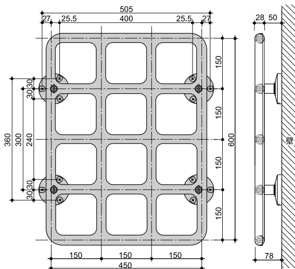
基本的な寸法 (単位mm) (プラスチック成形品につき多少の誤差があります。)
